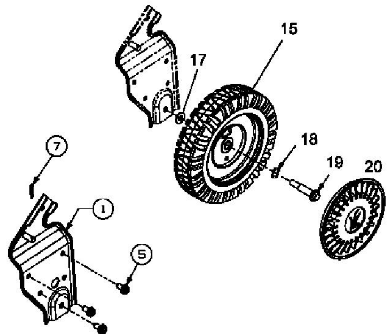
HINTERRÄDER/ REAR WHEELS
