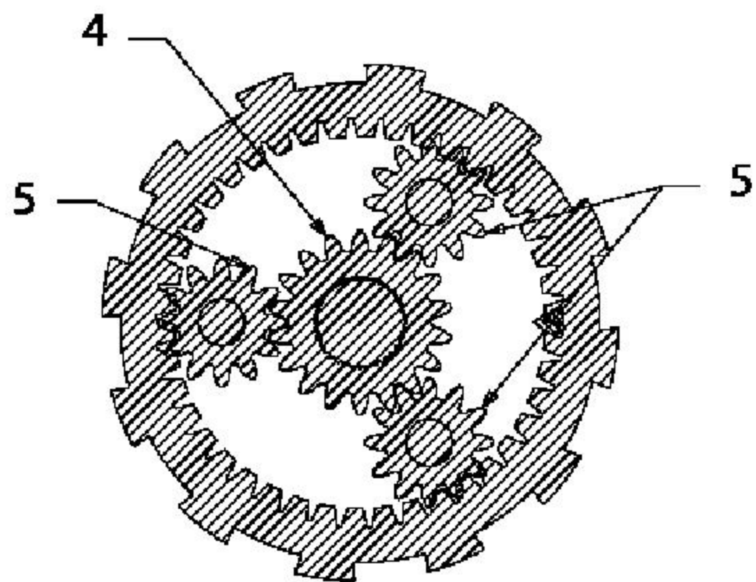
Schnitt B - B Section B - B
