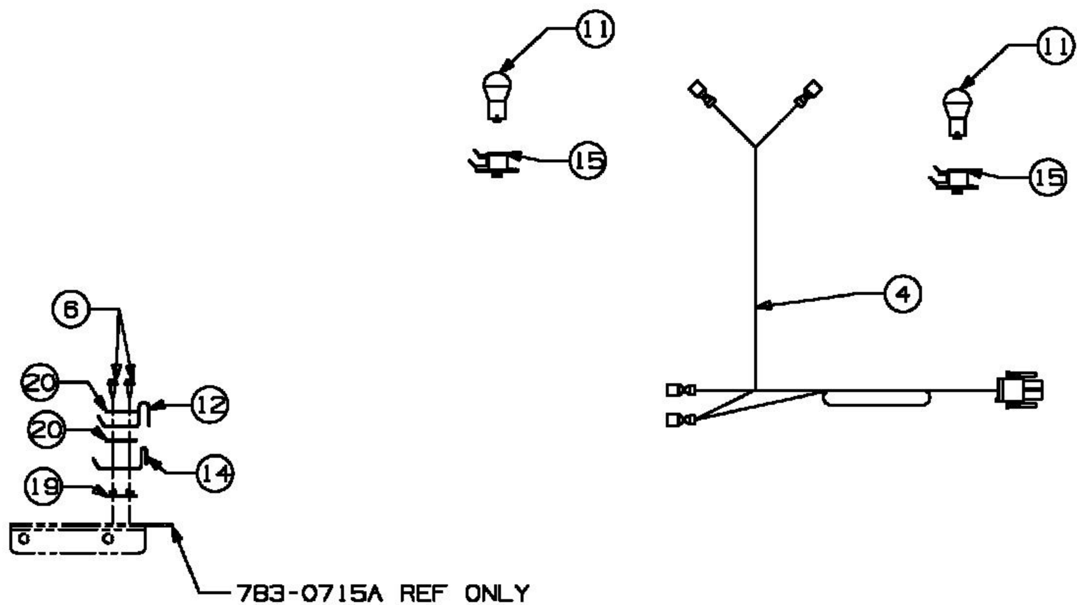
Sitzschalter / Seat Switch
