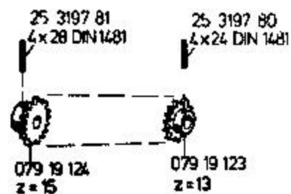
Art Nr 2627 09 Austauschkettenradsatz (von 3,6 km/h auf 4,15 km/h)
